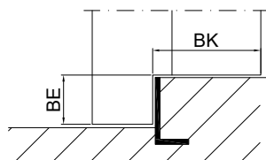
Klinkung bei bestehender Schwelle BE ..... x BK .....
