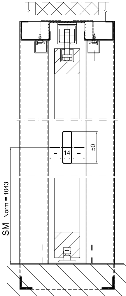
Riegelkasten Art. 84701
