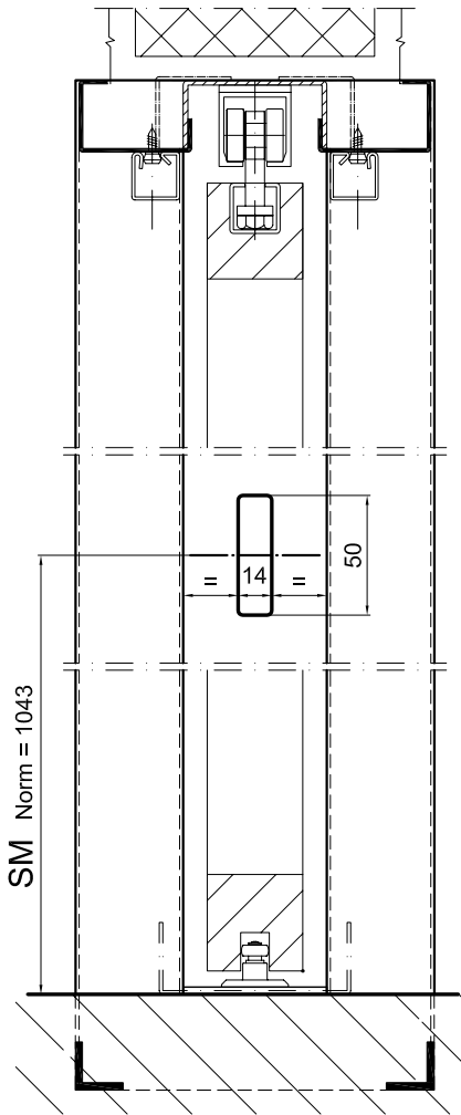
Spez. Riegelkasten
