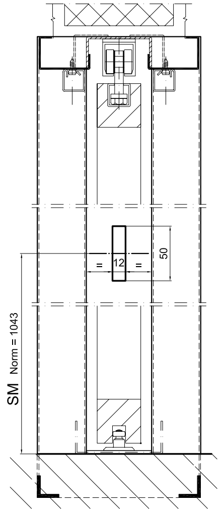
Riegelkasten Art. 84701
