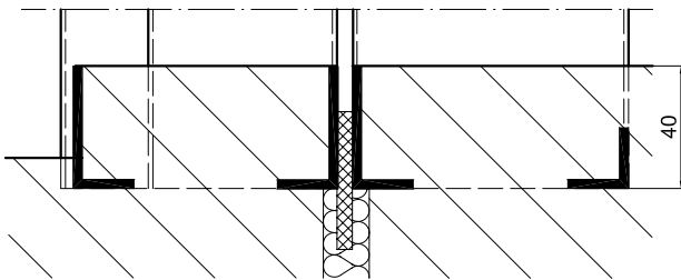
Beispiel: Schwelle Typ S Exemple: Seuil Type S
