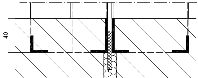
Beispiel: Schwelle Typ O Exemple: Seuil Type O
