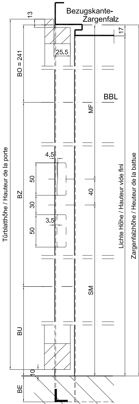
Schwelle /Seuil Typ O
