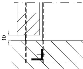
Schwelle/Seuil Typ PVU od. PV
