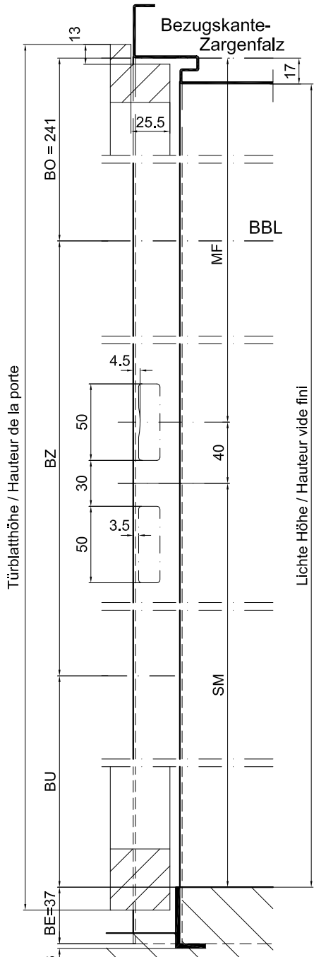
Schwelle/Seuil Typ DB
