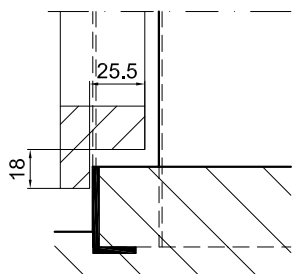
Schwelle/Seuil Typ SB
