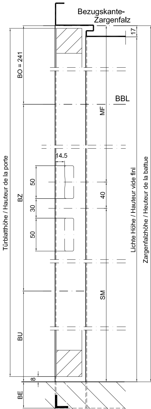
Schwelle /Seuil Typ O
